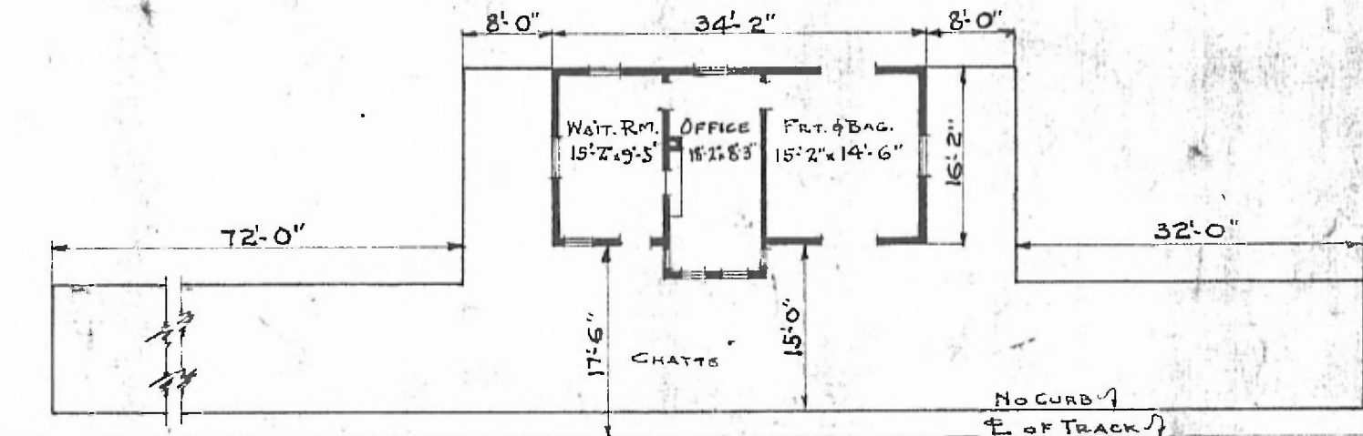
FLOOR PLAN SCALE: \frac{1}{16}'' = 1'-0''
